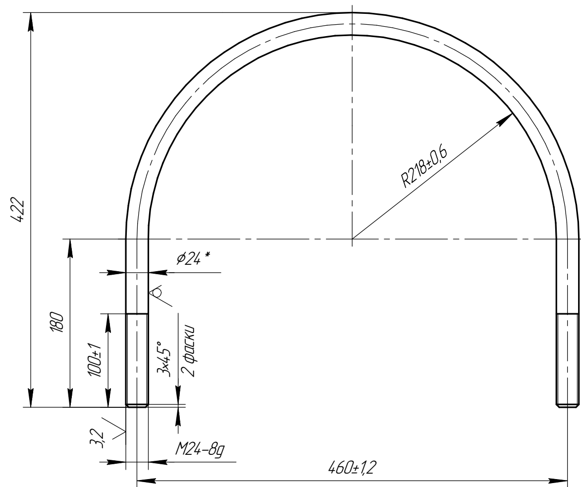
Дет. поз. 5
