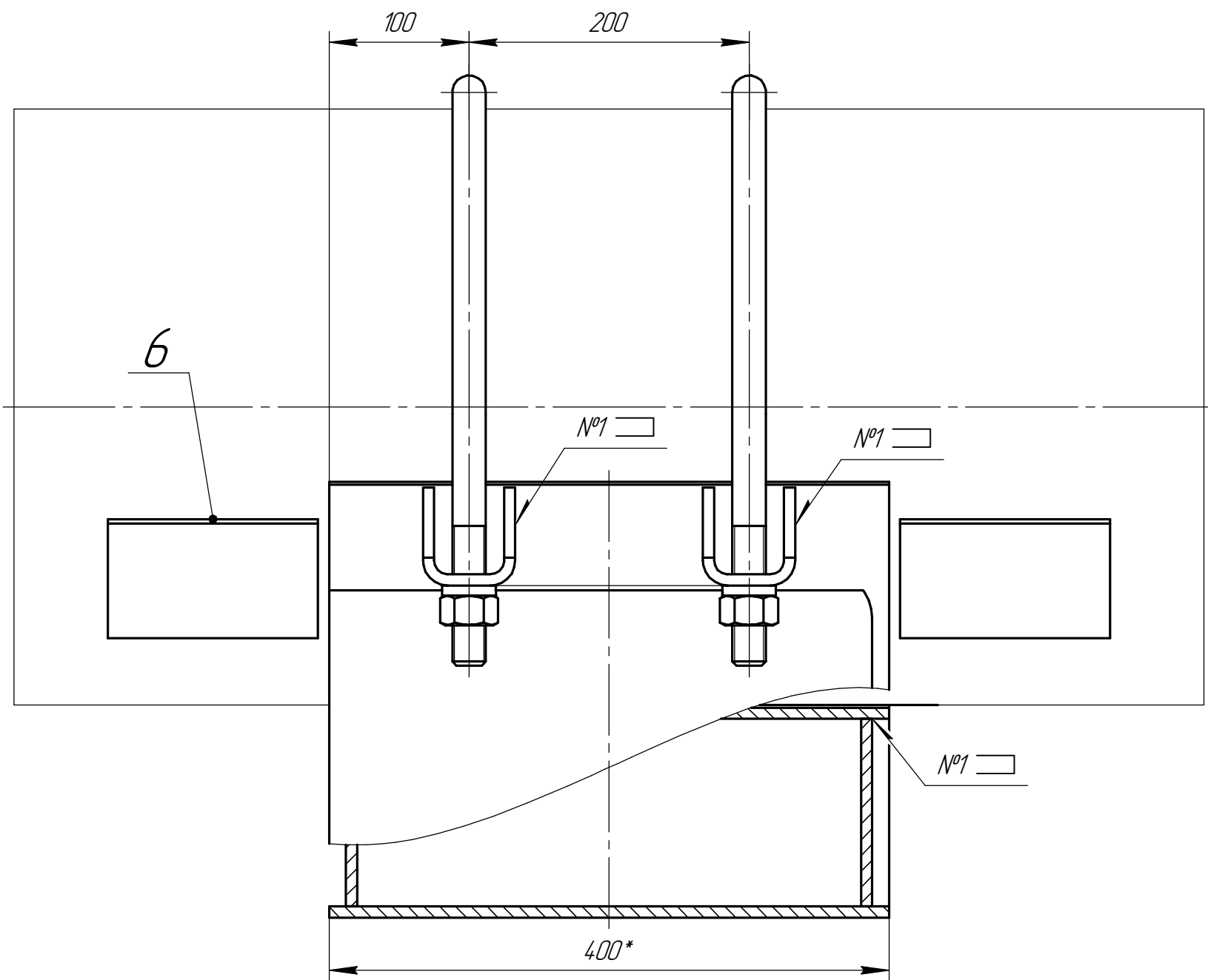
Дет. поз. 6 (1:2)
