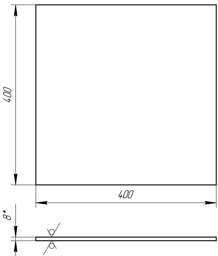
Дет. поз. 2
