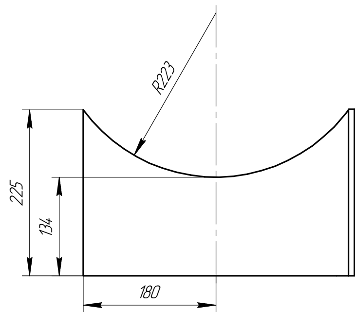
Дет. поз. 1
